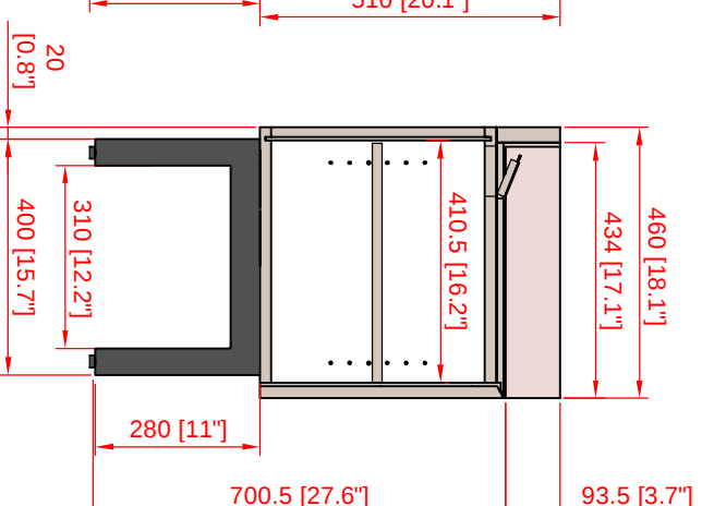
SECCIÓN B-B'
