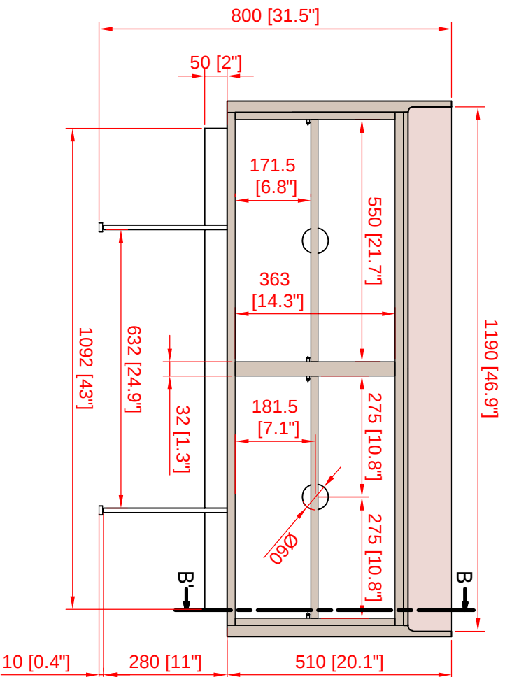
SECCIÓN A-A'
